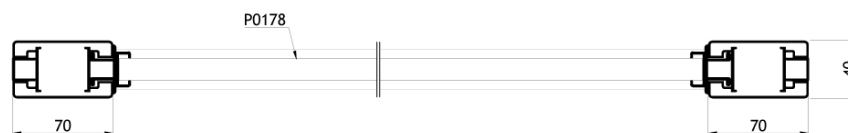
Section horizontale
