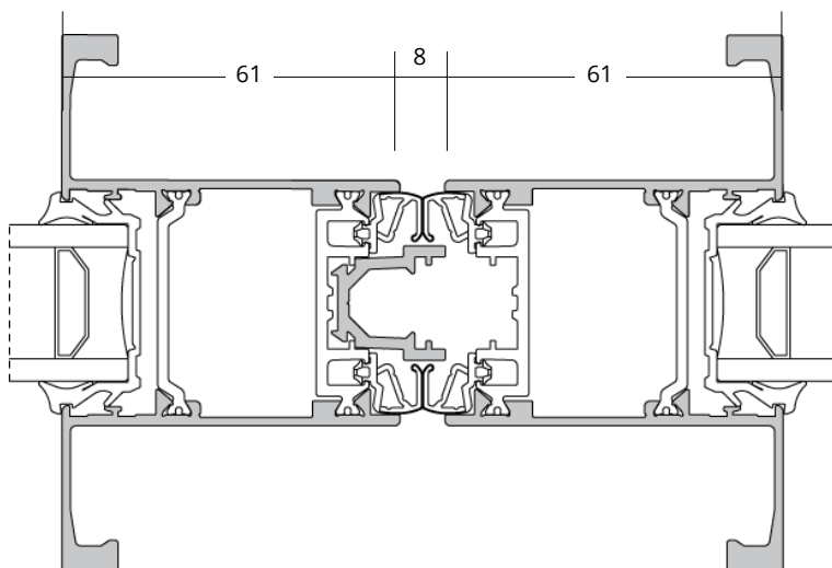
Montant double renfort et serrure H.>2250
