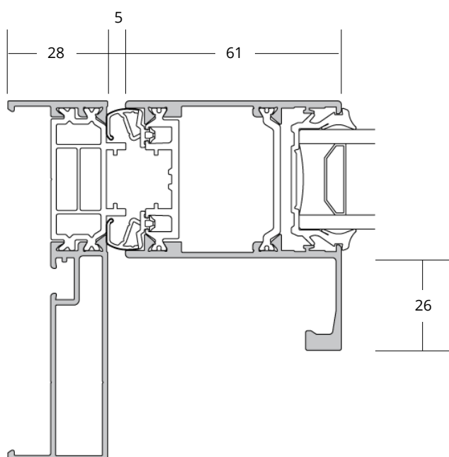
Montant renforcé large Cas serrure jusqu'à H.2250
