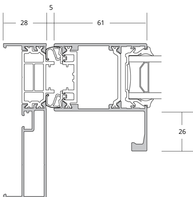
Montant renforcé large Cas serrure jusqu'à H.2250
