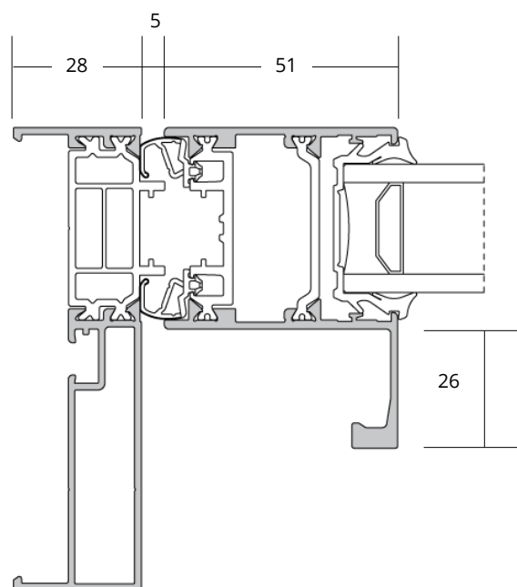
Montant renforcé H.>1650 jusqu'à 2250
