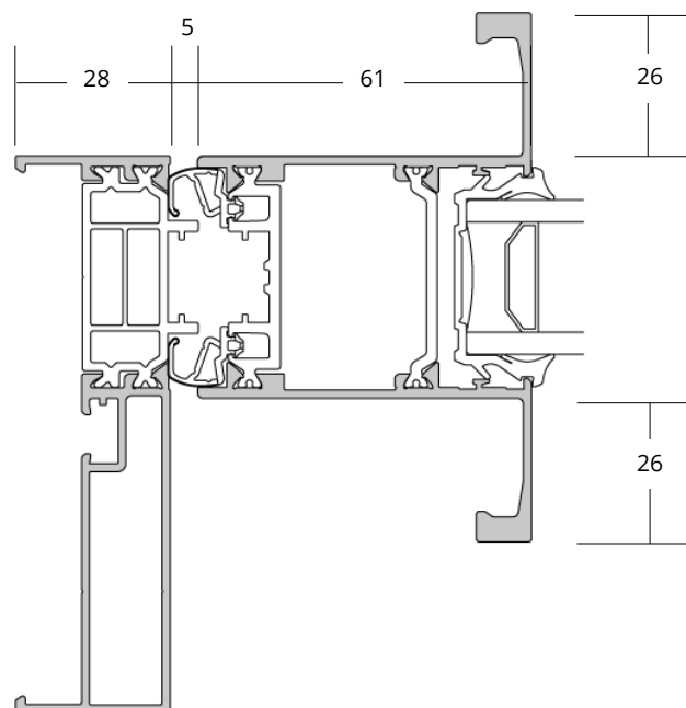
Montant double renfort et serrure H.>2250
