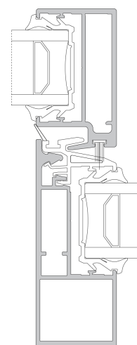
Montant double renfort et serrure H.>2250
