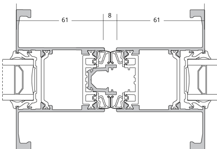
Montant double renfort et serrure H.>2250
