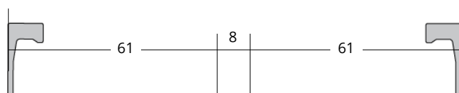
Montant double renfort et serrure H.>2250
