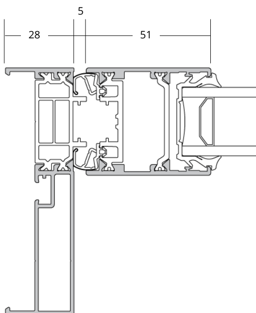
Montant simple H.<1650
