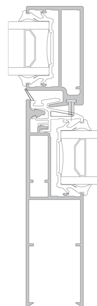
Montant double renfort et serrure H.>2250
