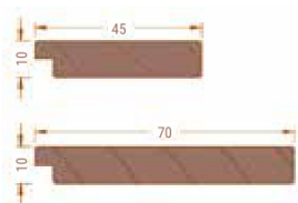
Couvres-joints plats intérieur et extérieurs
