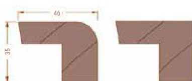
Cornière ext. Réno (option)
